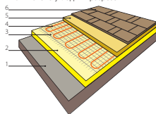
Рис. 7. Схема укладки в разрезе
