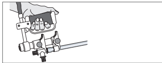
Рис 4-9 Соединение, вставленное в инструмент.
