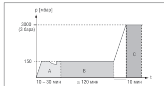
Рис. 17.2-9 Диаграмма пневматического испытания А Предварительное испытание (см таб. 17.2-1) В Основное испытание С Испытание нагрузкой
