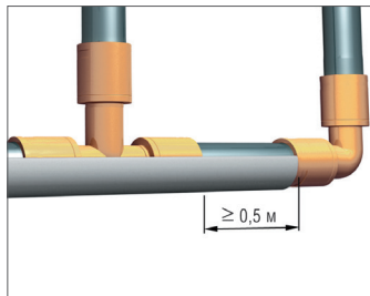
Рис. 9-4 Прокладка фиксирующего желоба поверх троек
