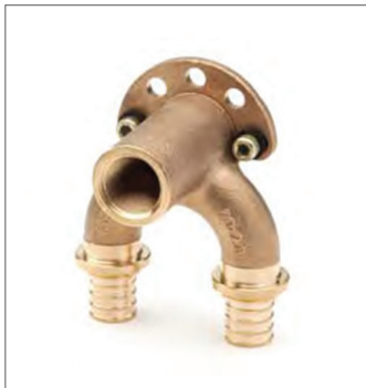
Рис. 17.2-2 Проточный угольник из бронзы
