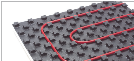
Система крепления труб на маты с фиксаторами Varionova
