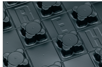
Рис. 15.5-14 Лицевая сторона мата с фиксаторами Varionova с шагозвукоизоляцией 30-2 снизу и теплоизоляцией 11 мм снизу
