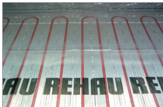
Рис. 15.6-1 Система укладки труб на теплоизоляционных матах TS-14
