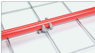
Рис. 15.5-27 Крепление труб 20 мм вдоль основания клипсы
