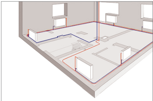
Рис. 14.1-3 2-х трубная горизонтальная полупная
